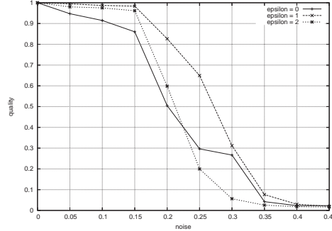
FIG. 1 – Qualité des ET-4-ensembles fermés extraits avec \epsilon \in \{0, 1, 2\}
