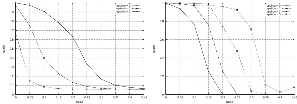
(a) Espace de taille 16 \times 16 \times 16 cachant des 3-ensembles de taille 4 \times 4 \times 4
