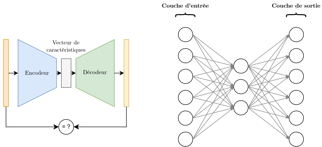
(a) Schéma de l'architecture globale d'un auto-encodeur.
