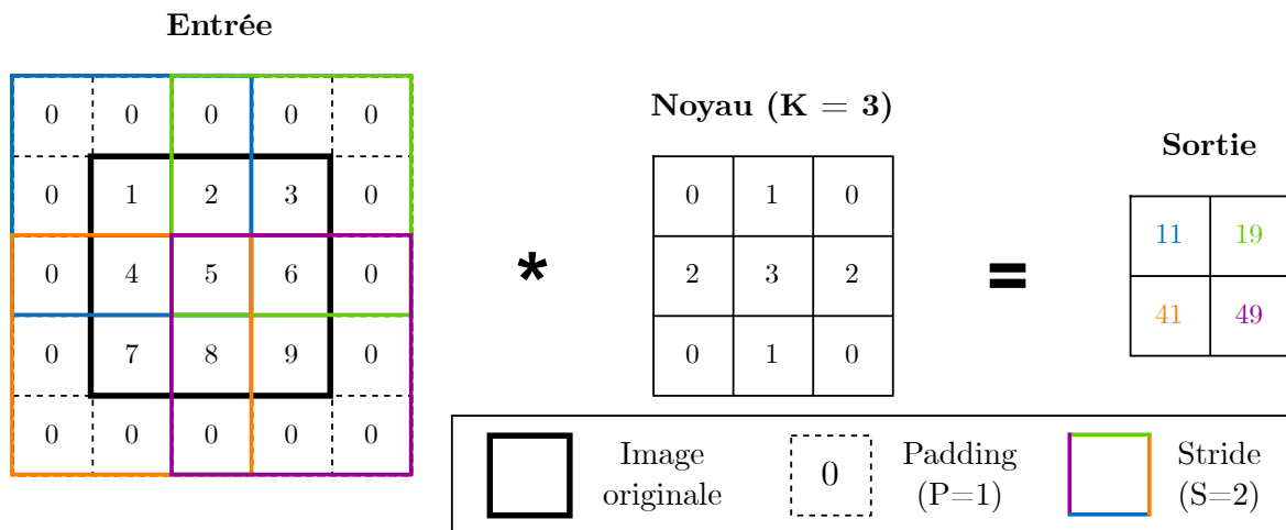
FIGURE 2.4 – Illustration de l'application d'une convolution, avec K = 3 , P = 1 et S = 2
